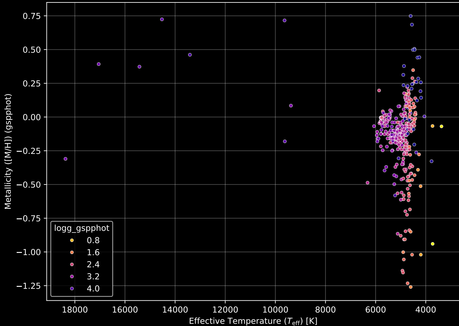
APOGEE DR17 Field: [240-08] Stellar Population Parameters (n= 416)
